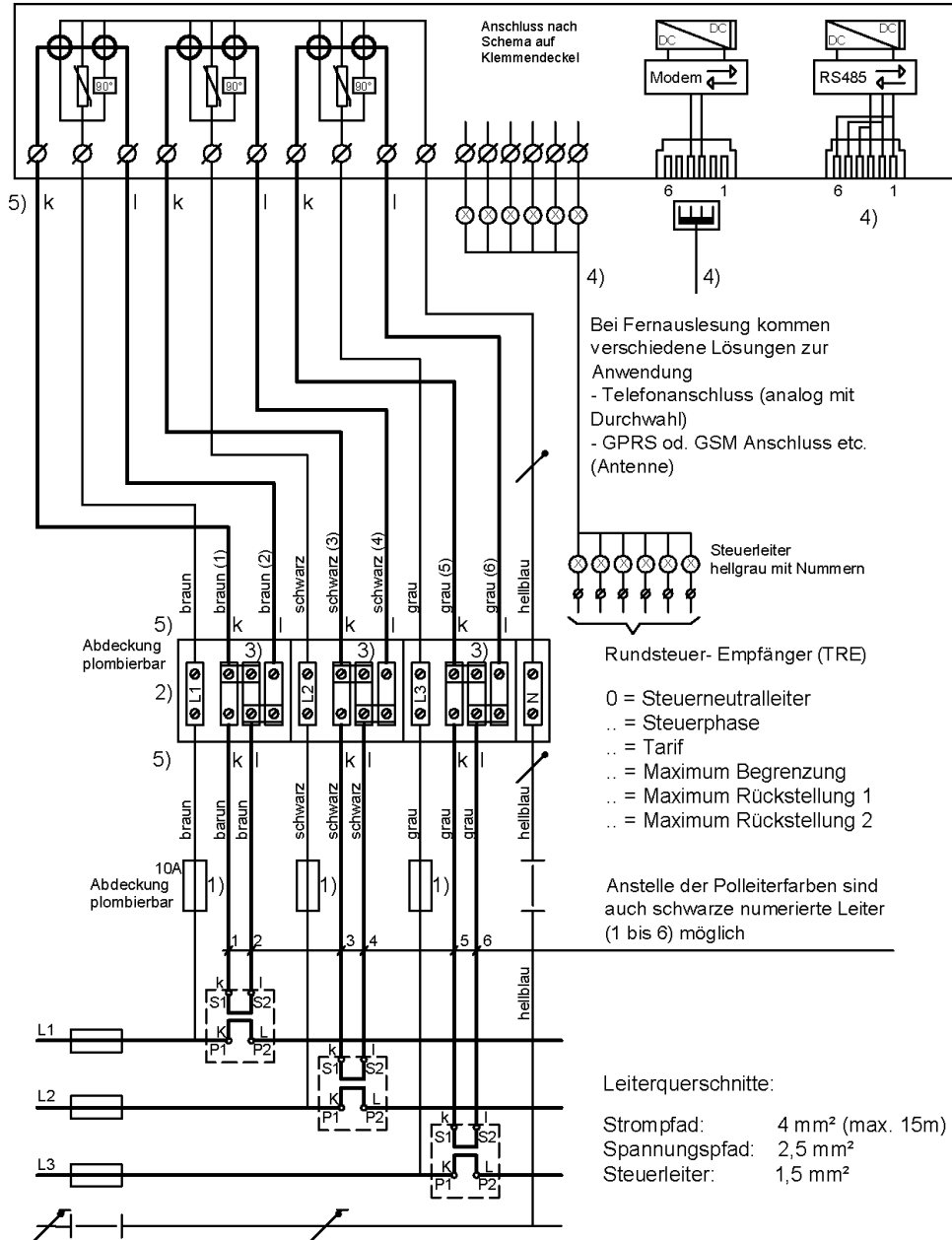
Wirk.-/Blindenergiezähler kombiniert
